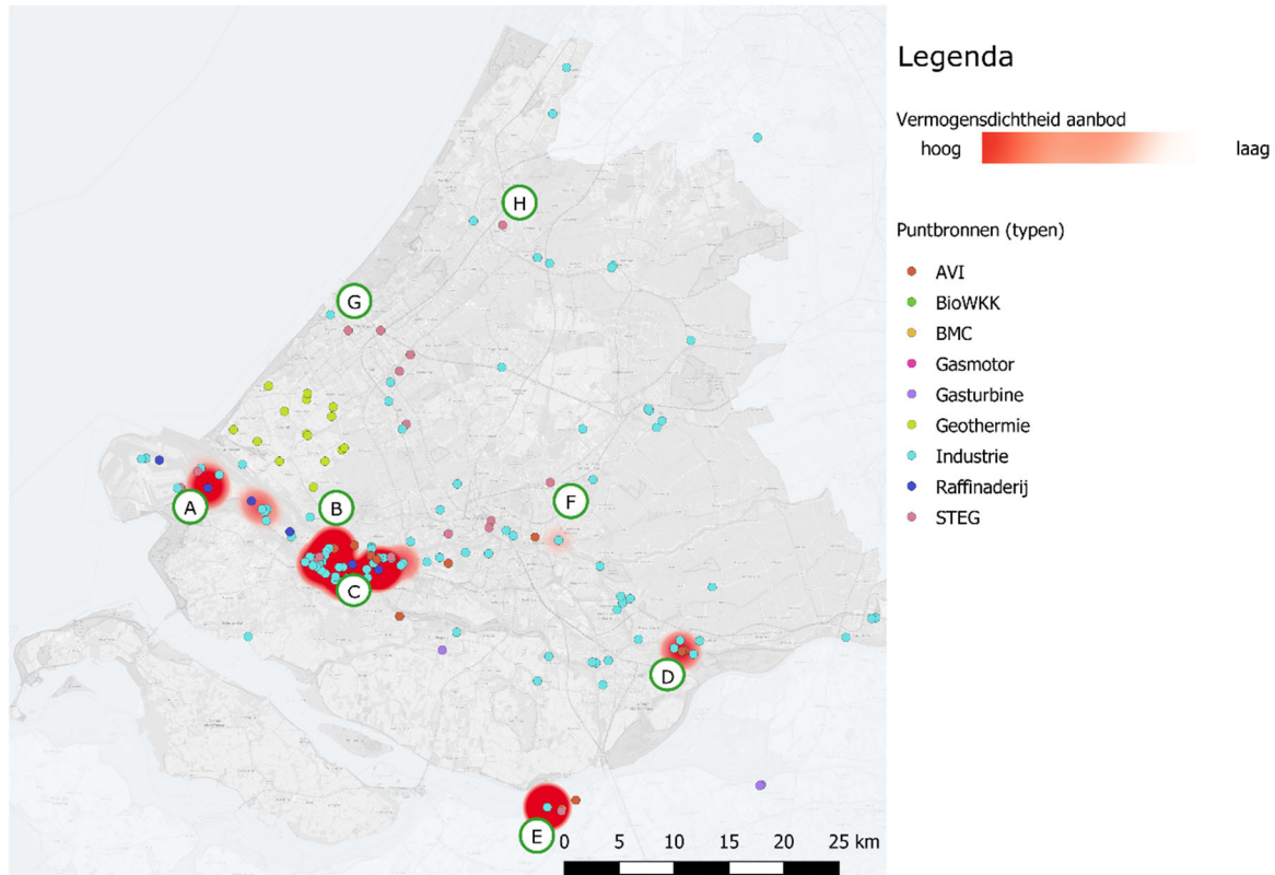
Figuur 25. Bronnen van restwarmte. De "heatmap" geeft de vermogensdichtheid aan.
